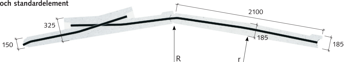
Tvärsnitt av spännelement och standardelement
